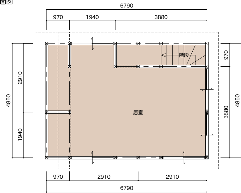
■2F平面図
