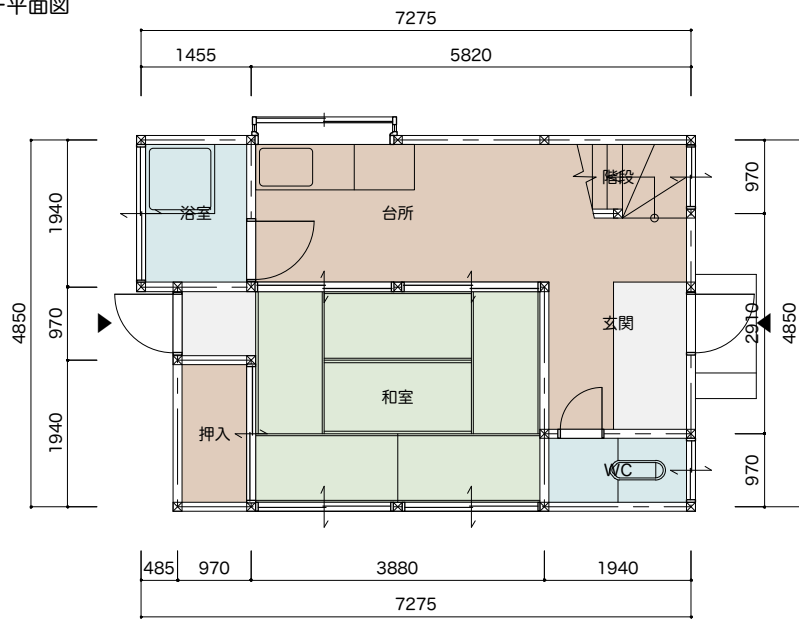
■1F平面図
